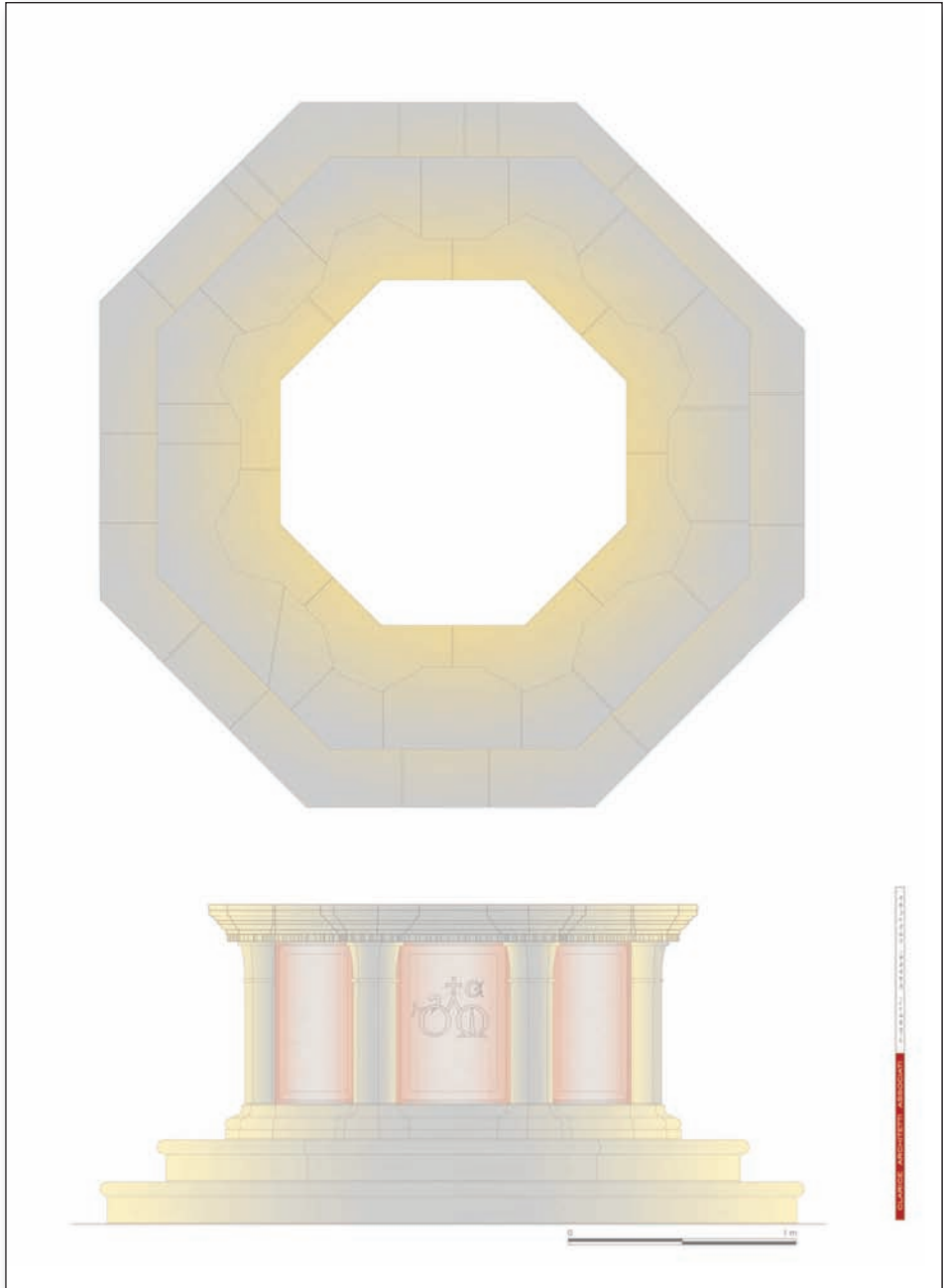
Pianta e prospetto della Vera di pozzo realizzata dall'Architetto Edi Grassi
